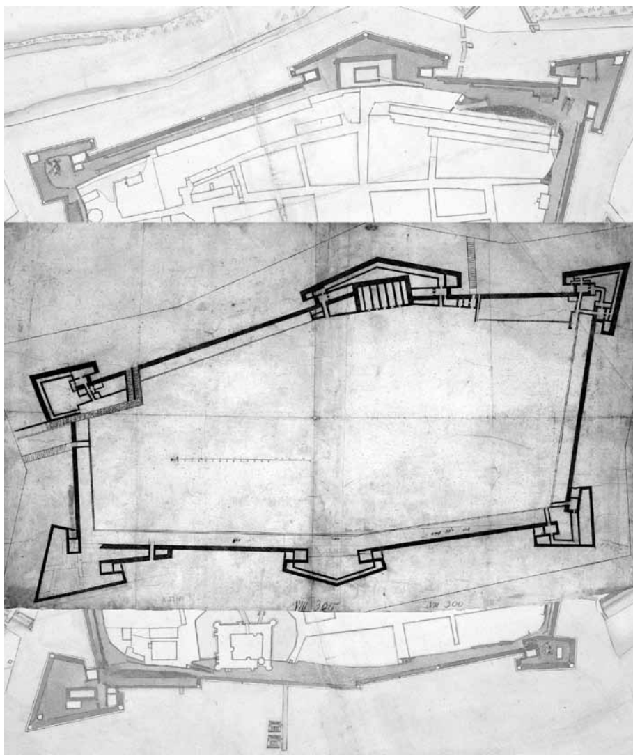
Il. 9. Niewątpliwie najstarszy, jednak niedatowany, rysunek umocnień Kostrzyna (zbiory Działu Kartograficznego Biblioteki Państwowej w Berlinie, sygn. X 22180; pośrodku) łączy cechy inwentaryzacji i projektu. Dzieła na północno-wschodnim boku warowni (u góry) dość dokładnie odpowiadają mianowicie formą przedstawionym na planie Jakuba Holsta z 1650 r. (il. 8), podczas gdy dzieła nad Odrą (u dołu) znacznie od rzeczywistości zrealizowanych odbiegają formą – narzuca się wniosek, że w momencie kreślenia planu te pierwsze były już gotowe lub bliskie ukończenia, podczas gdy drugie były dopiero projektowane, a zrealizowane zostać miały ostatecznie tylko po części (bez środkowego bastionu) i przybrać odmienne formy. Przyjmujemy, że plan wyjść mógł jeszcze spod ręki Chiaramelli, a więc powstałby przed 1578 r.
