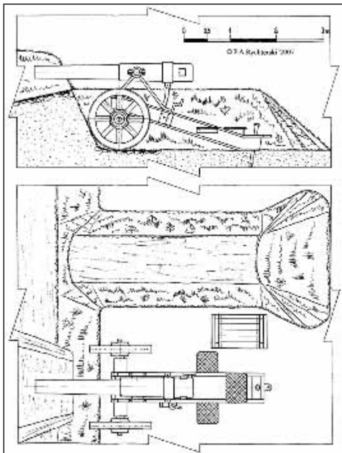
Abb. 6: Kanonenstand mit einer schweren Feldkanone, Muster 1872, Kaliber 15 cm, auf dem Artilleriewall. Abb. oben: Profil des Kanonenstandes, Ansicht des Querbalkens und der Kanone von der Seite; Abb. unten: Abschnitt des Kanonenstandes, die Kanone und der Querbalken - Ansicht von oben.
