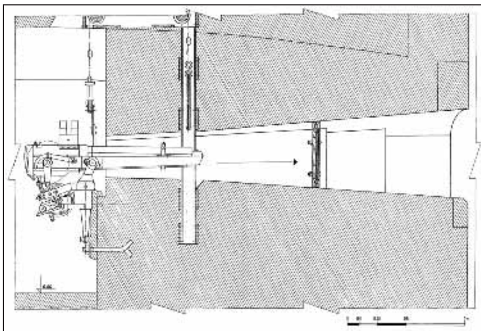
Rys. 11: Przekrój pionowy podłużny strzelnicy artyleryjskiej w kaponierze fortu. W świetle otworu widoczna armata rewolwerowa Hotchkiss/Gruson, kaliber 3,7 cm.
