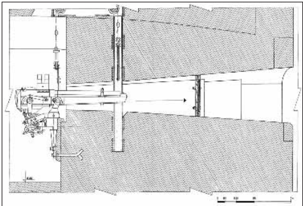
Abb. 11: Längsausschnitt der Artillerieschießbank in der Kaponniere des Fortes. In der Öffnung eine Revolverkanone sichtbar, Typ Hotchkiss/Grusson, Kaliber 3,7 cm.
