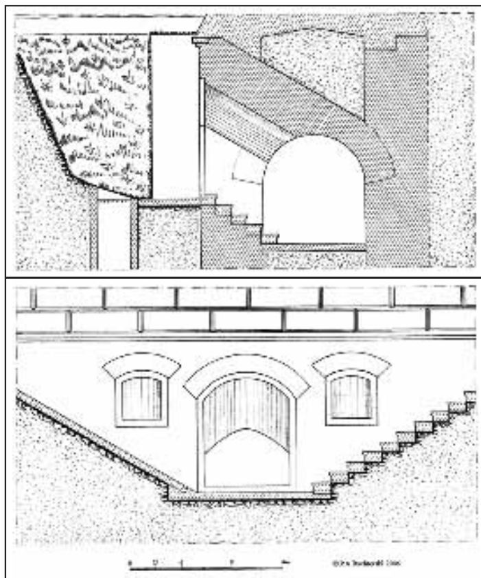
Rys. 15: Lewa kaponiera barkowa: rysunek górny - przekrój pionowy poprzeczny schronu pogotowia na wale piechoty; rysunek dolny - fasada schronu i wybieżnia na wale piechoty.
