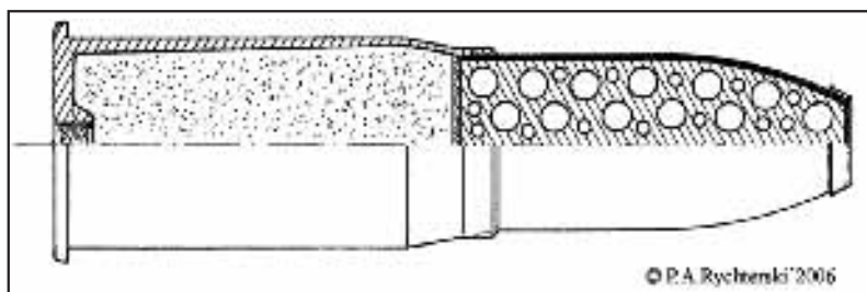
Rys. 10: Nabój kartaczowy, kaliber 3,7 cm, wersja A, do armaty rewolwerowej Hotchkiss/Gruson. Skala 1:1.
