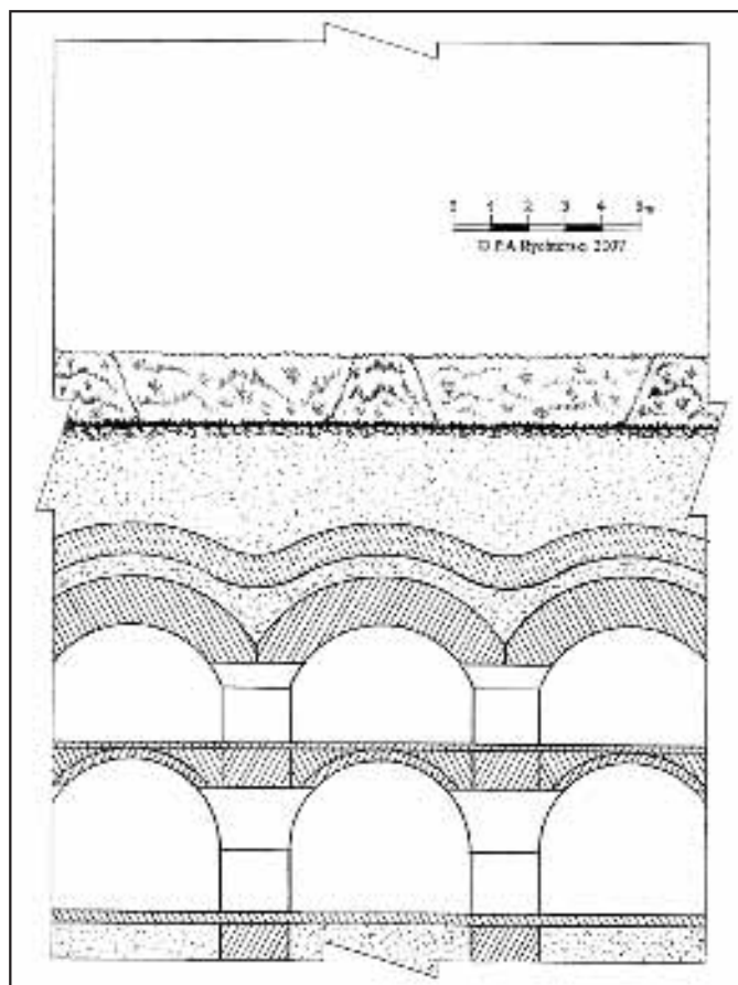
Abb. 18: Längsausschnitt eines Fragmentes der vorderen Kaserne. Oben: Kanonenstand auf dem Artilleriewall sichtbar.
