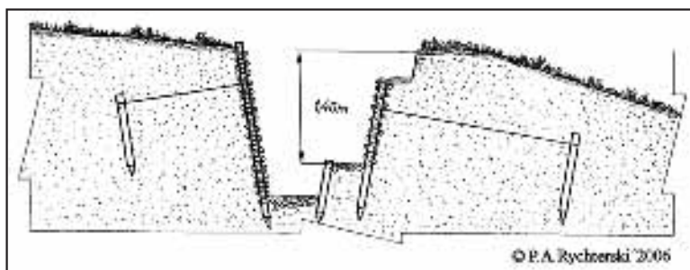
Rys. 13: Wałowa ławka strzelecka.
