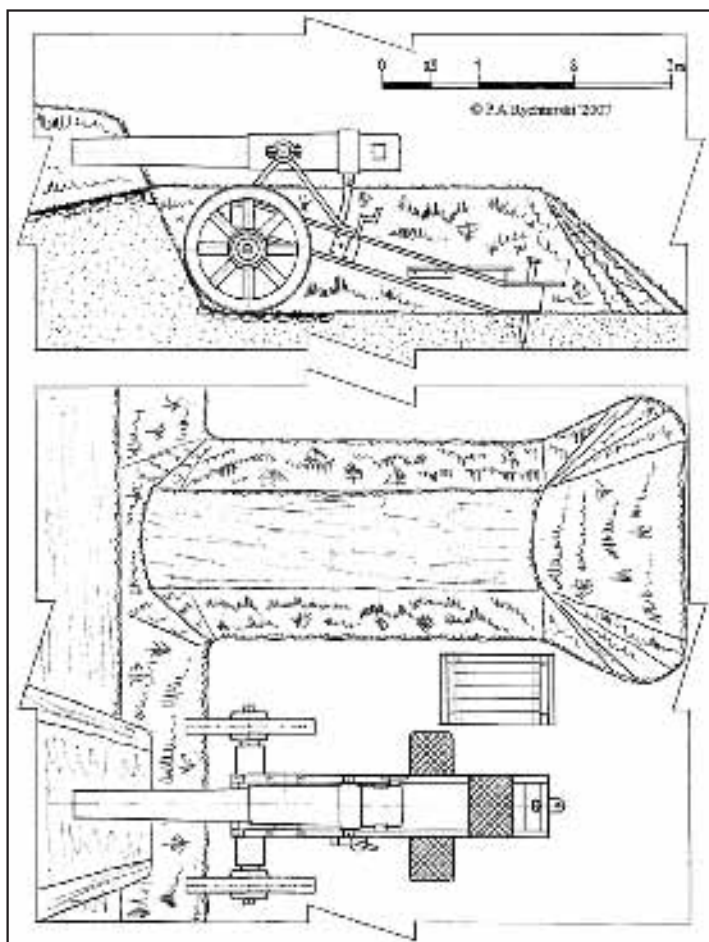
Rys. 6: Działobitnia z ciężką armatą połową wzór 1872, kaliber 15 cm na wale artylerii. Rysunek górny - profil działobitni, widok poprzecznic i armaty z boku; rysunek dolny - fragment działobitni, armata i poprzecznica - widok z góry.
