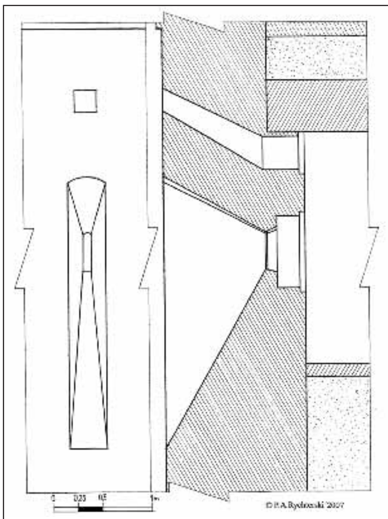
Abb. 14: Außensicht und Queraufriss der Schießbank der Infanterie in den Kaponieren des Fortes.
