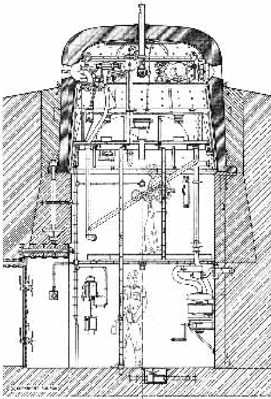
Rys. 6 Sześciostrzelnicowa kopuła 20P7
